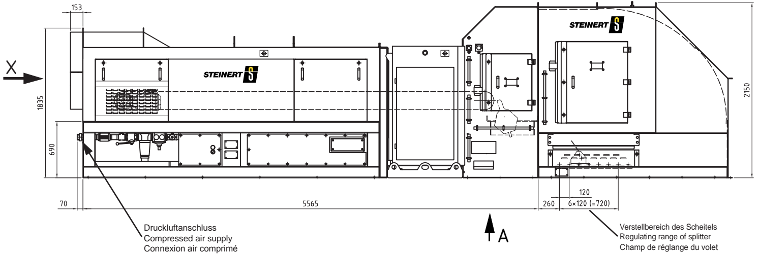
Ansicht A View A Vue A
