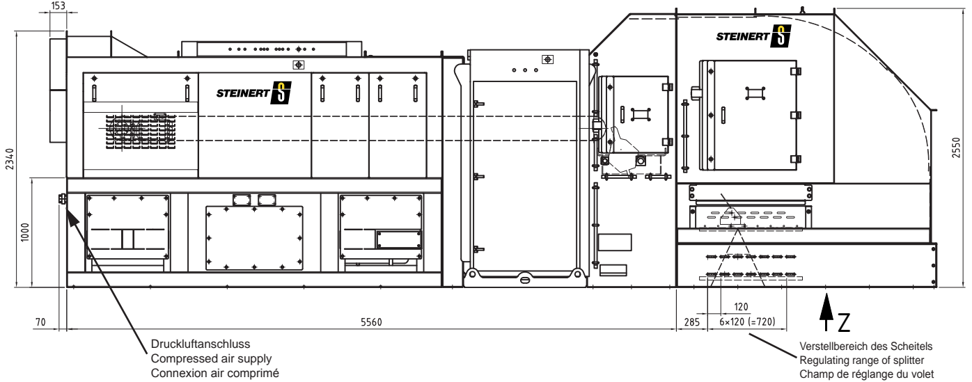
Ansicht Z View Z Vue Z
